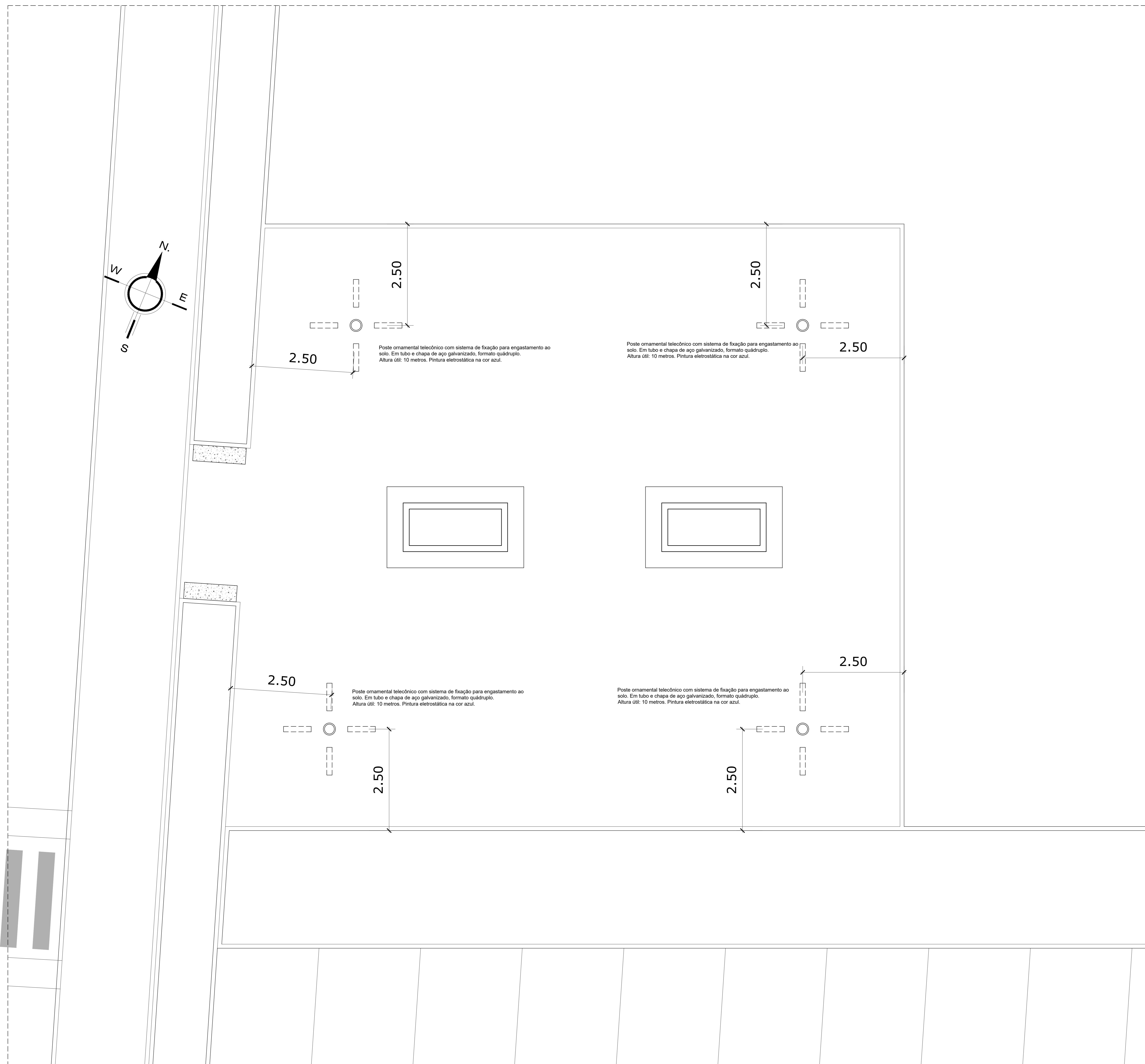
PLANTA DE LOCAÇÃO DE POSTES ESCALA 1/50
