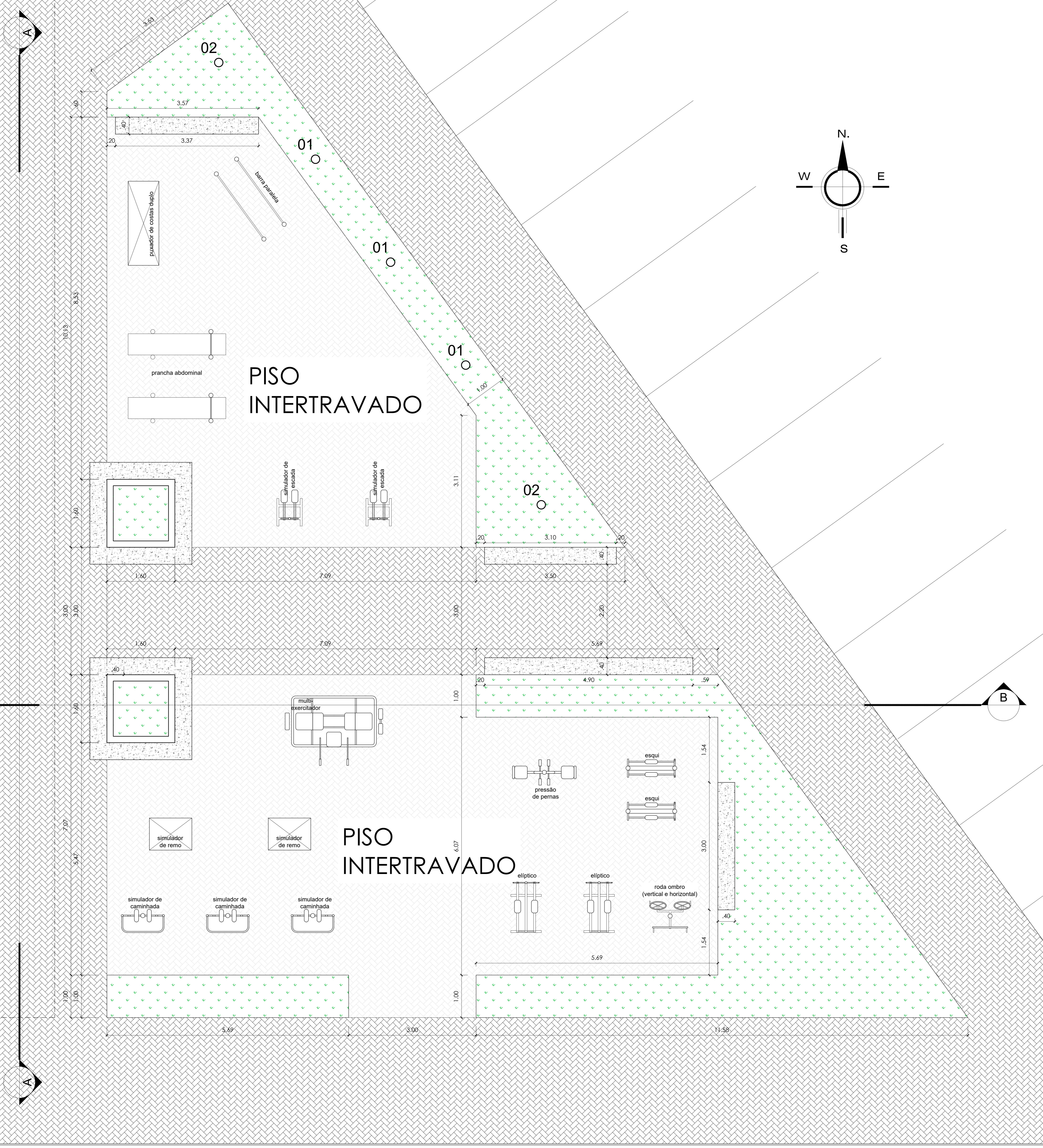
PLANTA BAIXA ESCALA 1/50
